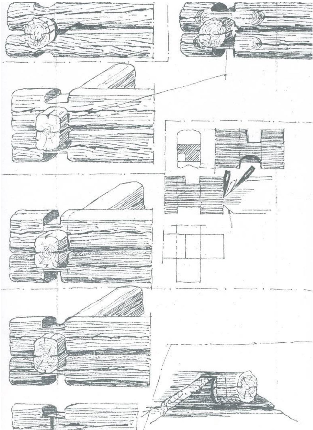
Gamla knutar och en del andra detaljer vid liggtimring
